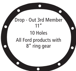
FORD 8"
