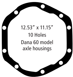
DANA 50/DANA 60
